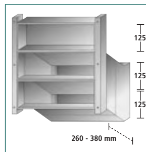
BDT Mauerdurchwurfkasten 1-teilig Tiefe ausziehbar
