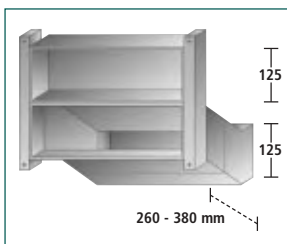
BDT Mauerdurchwurfkasten 1-teilig Tiefe ausziehbar
