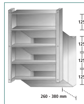
BDT Mauerdurchwurfkasten 2-teilig Tiefe ausziehbar
