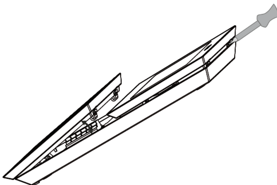
Bild 3: Zusammenbau / Demontage
