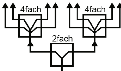
Bild 10: Verteiler Kaskadierung
